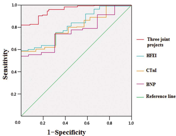
图1 HFEI 以及血清 cTnI、BNP 联合预测 MACE 效能的 ROC 曲线
